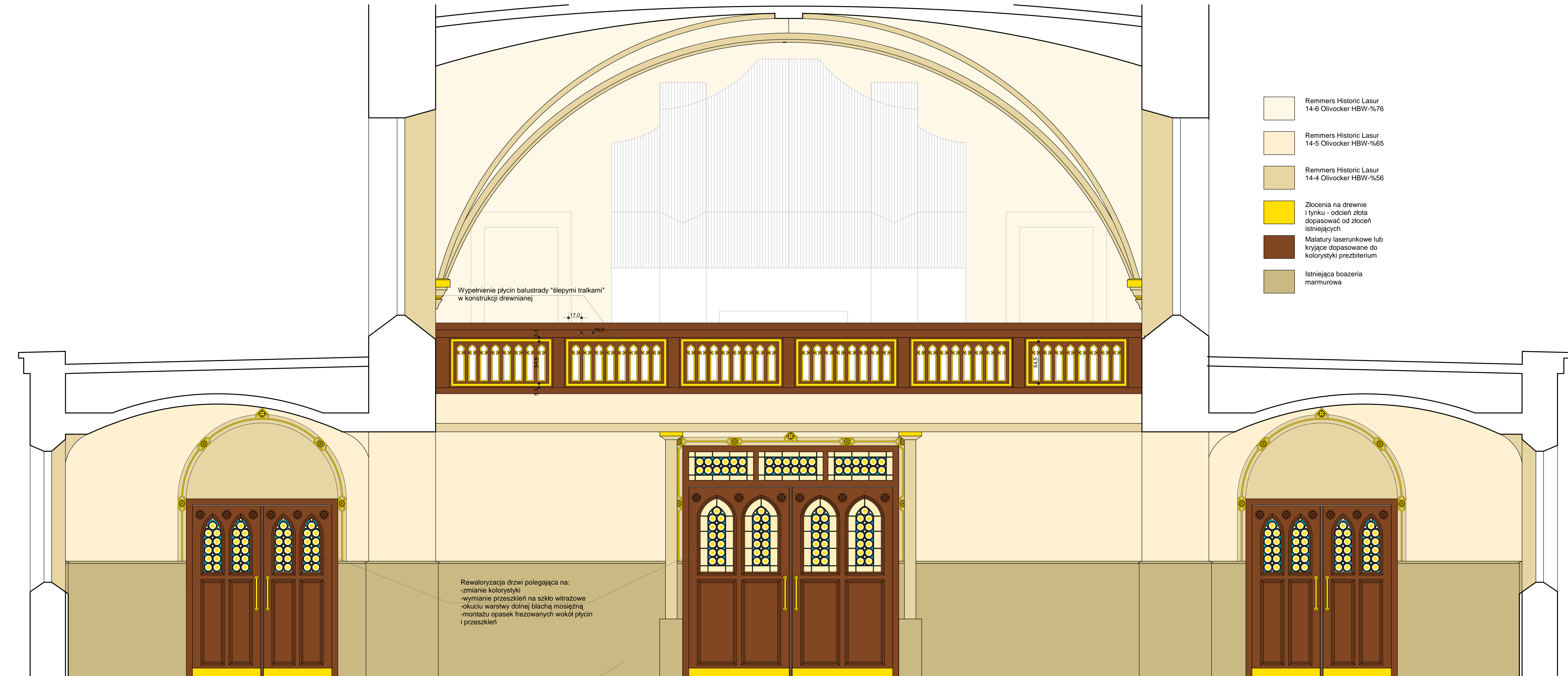
WIDOK ŚCIANY TYLNEJ (CHÓR) 1:25
